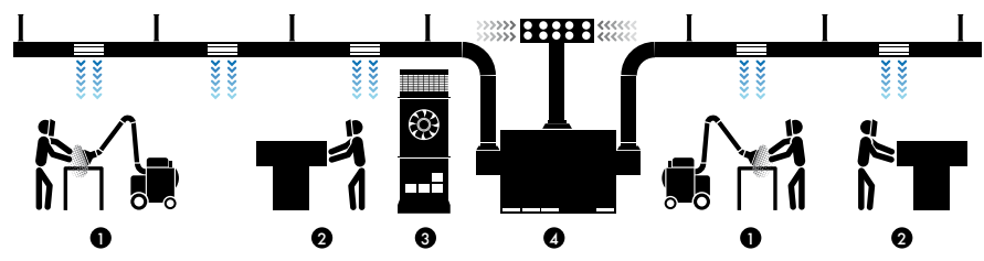
1. Aspirador móvil. 2. Mesa de aspiración. 3. Torre de filtración. 4. Sistema de aspiración ambiental.
