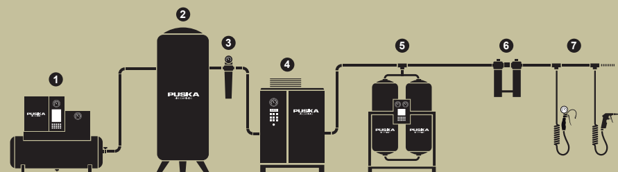
1. Compresor de tornillo 2. Depósito de aire 3. Filtro 4. Secador frigorífico 5. Secador de adsorción 6. Separador agua/aceite 7. Aplicadores aire comprimido.
